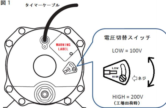
図1 タイマーケーブル
