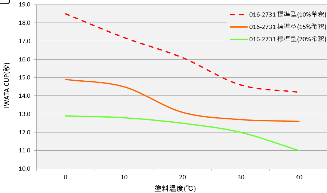
温度-粘度曲線 [ 073-8204 ハイロックDX ホワイト ]
