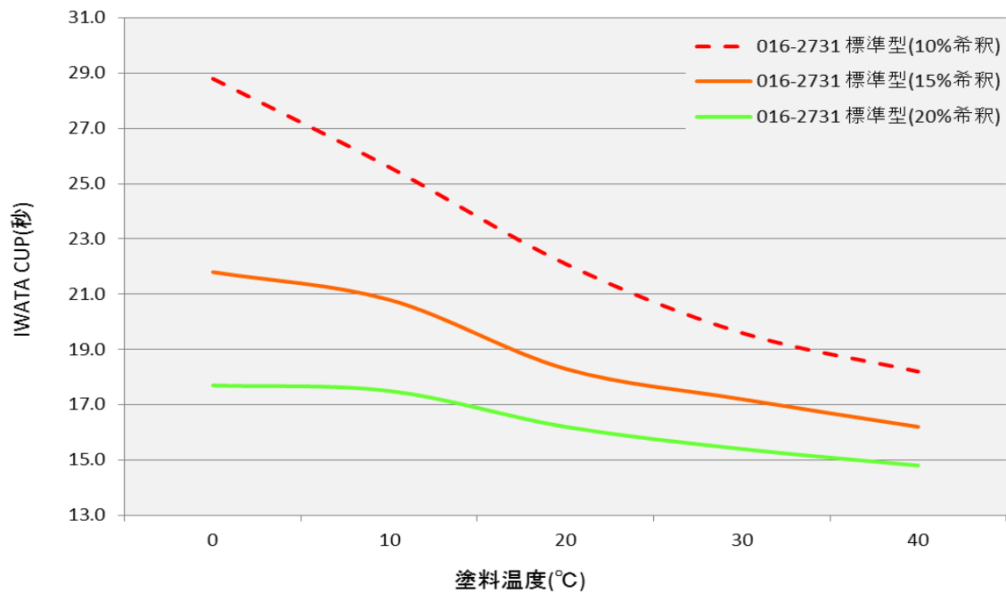
温度-粘度曲線 [ 073-8234 ハイロックDX ブラック ]
